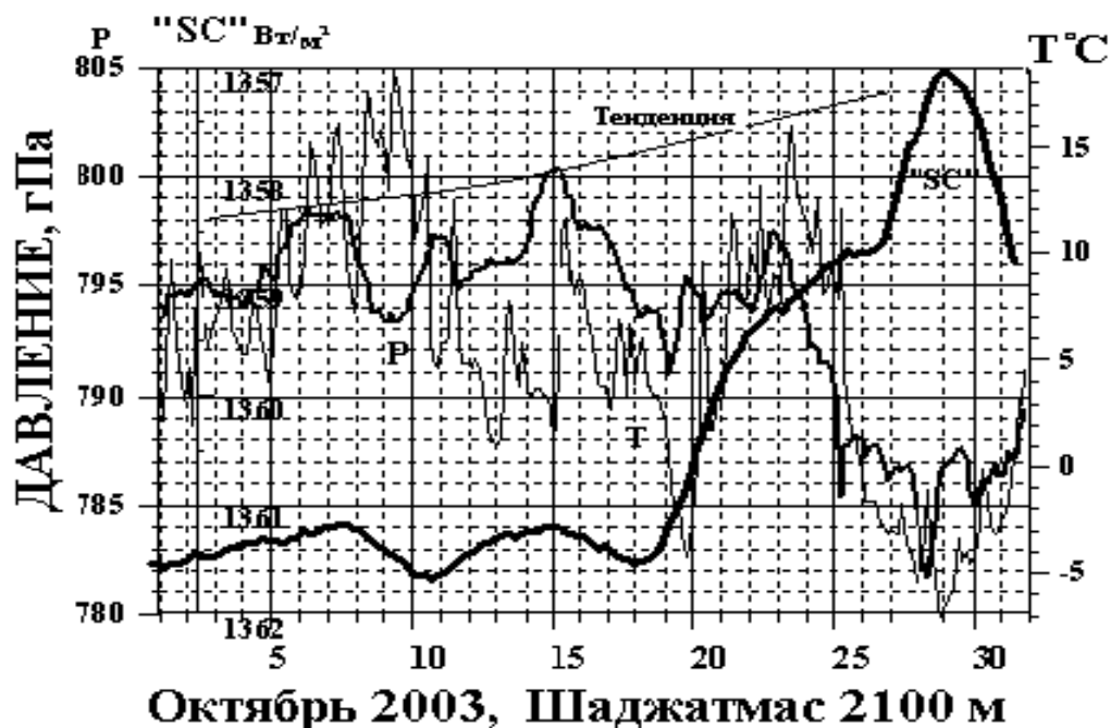
Рис.2. Изменения приземного давления P и температуры воздуха T представлены по трехчасовым данным метеостанции Шаджатмас для октября 2003 года совместно с изменениями солнечной постоянной в обращенной шкале ее значений. “Спокойный” ход синоптических вариаций в первой половине месяца нарушается в последующие недели, по-видимому, под воздействием внешнего силового фактора.
