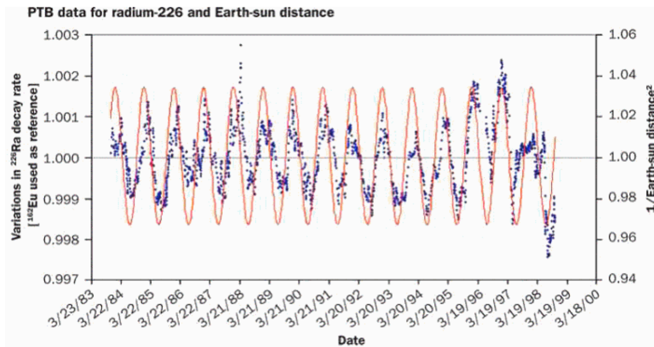
Рис. 4. Представлена связь (для 15-ти летнего ряда непрерывных наблюдений [11]) изменений скорости распада р/а изотопа Ra 226 с относительными изменениями обратной величины квадрата расстояния между Землей и Солнцем ( 1/R^2 ). Следует отметить, что при очевидной тесной корреляции между упомянутыми параметрами, в некоторые периоды времени появляется фазовый сдвиг, а также тенденция к дополнительному увеличению скорости распада на периоде роста солнечной активности в 22 и 23 циклах (весенние максимумы 1988 и 1997 г). Наличие достоверной корреляционной связи во многом определяет характерные черты фактора, воздействующего на ядра изотопа (или, что не исключено, на активное вещество детектора), а именно: а) указывает на его внутри солнечное происхождение; б) на его полевой, а не корпускулярный характер; в) на то, что его поле имеет сродство с электромагнитным полем Солнца только по месту их генерации и по характеру их распространения в пространстве ( 1/R^2 ); г) воздействие нового (вихревого) фактора на активное вещество детектора излучений будет интегрироваться с его воздействием на ядра атомов; д) электромагнитное поле не оказывает какого-либо воздействия на вихревое поле, поскольку квант последнего нейтрален, но вихревое поле частично передает при встрече (например, в солнечном ветре) энергию импульса и хирального углового момента всем массовым частицам и, в первую очередь, электрону из-за его сравнительно небольшой массы.
